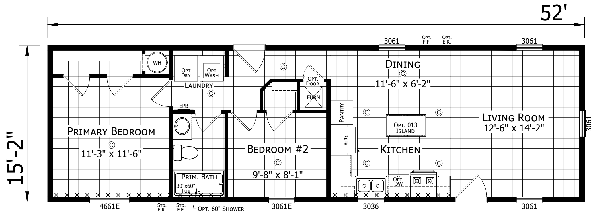
112AP-1652H21083 2 BEDROOM 1 BATH 52'-0" x 15'-2"
