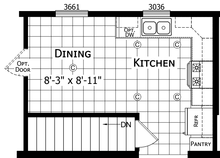
OPTIONAL STAIRWELL
