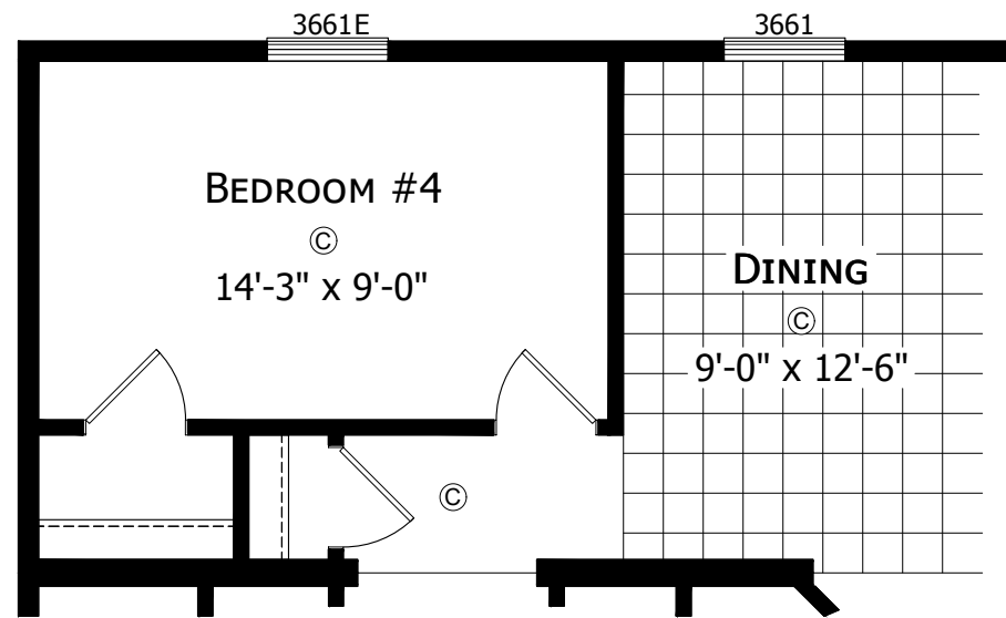
OPTIONAL BEDROOM #4
