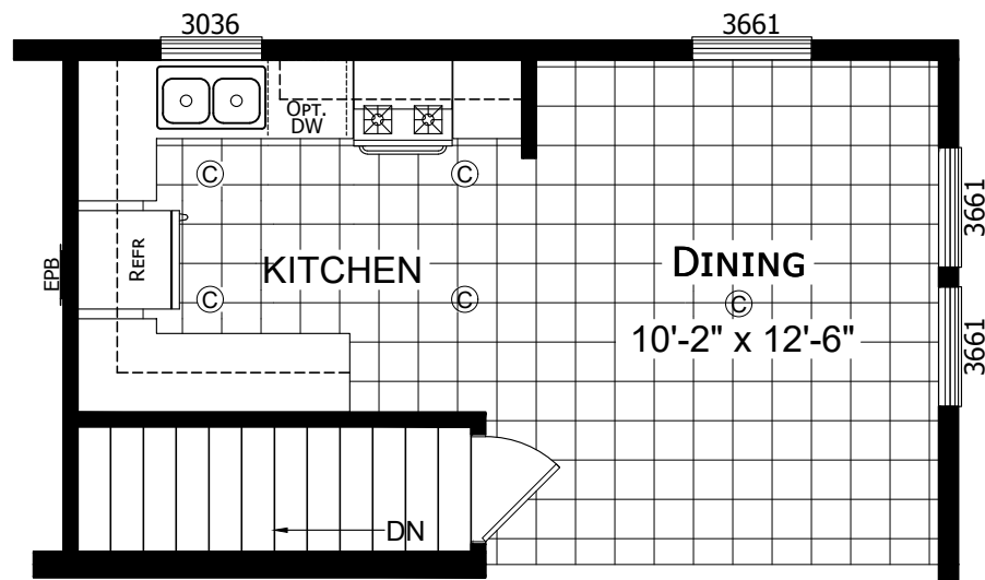
OPTIONAL STAIRWELL
