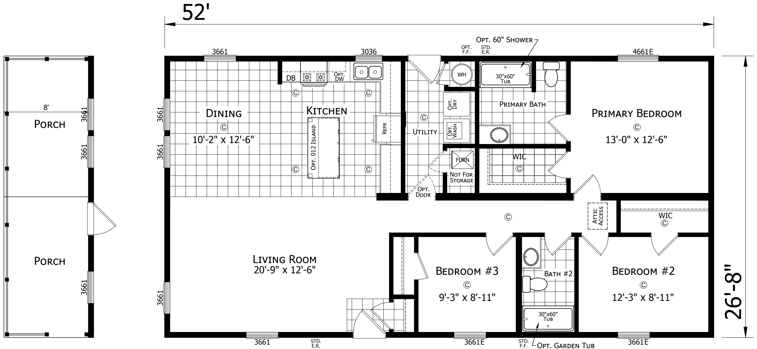
OPTIONAL PORCH
