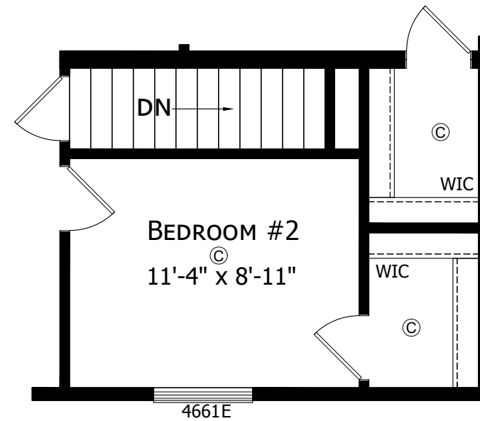
OPTIONAL STAIRWELL
