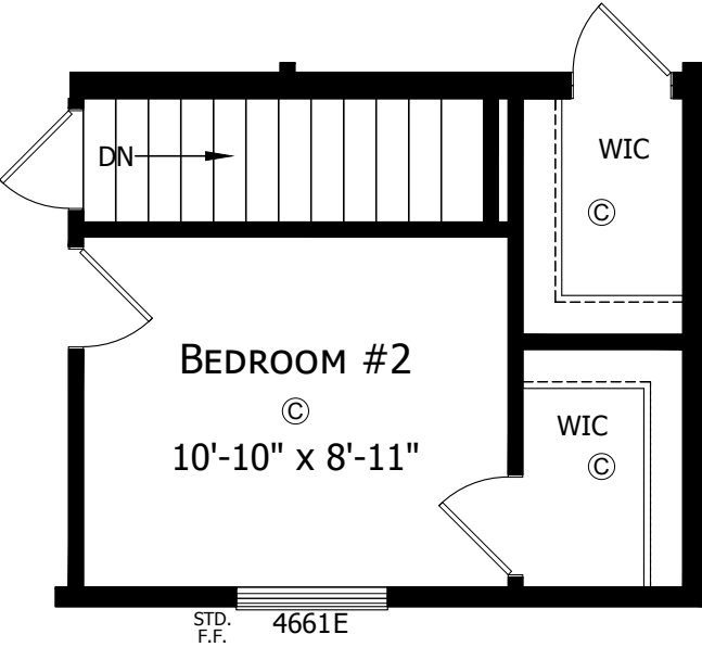
OPTIONAL STAIRWELL
