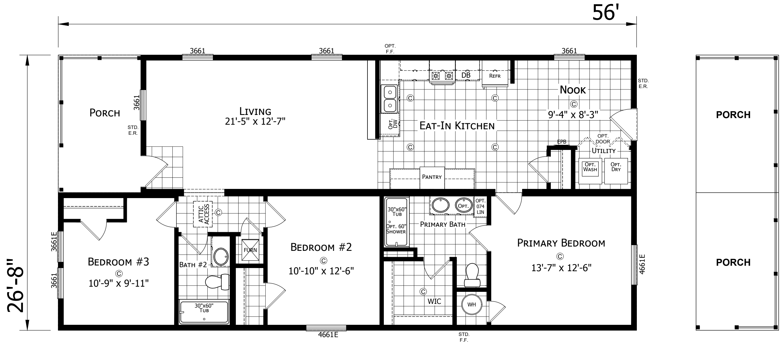
OPTIONAL 8' PORCH
