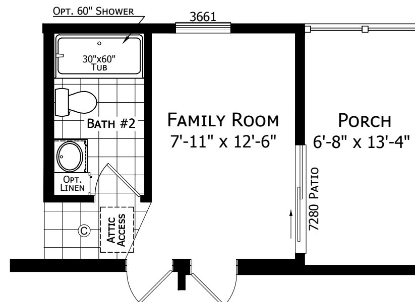
OPTIONAL 1/2 PORCH
