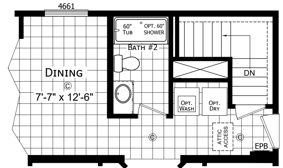
OPTIONAL STAIRWELL
