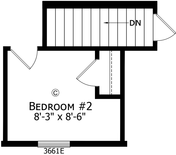
OPTIONAL STAIRWELL
