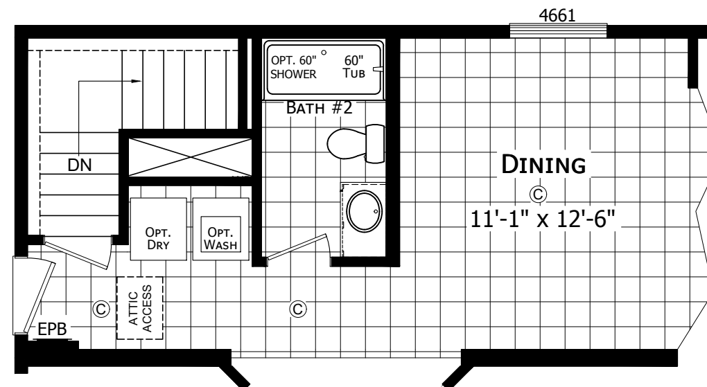
OPTIONAL STAIRWELL
