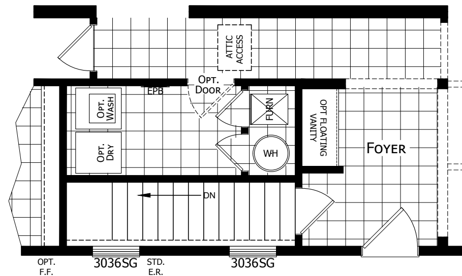
OPTIONAL STAIRWELL
