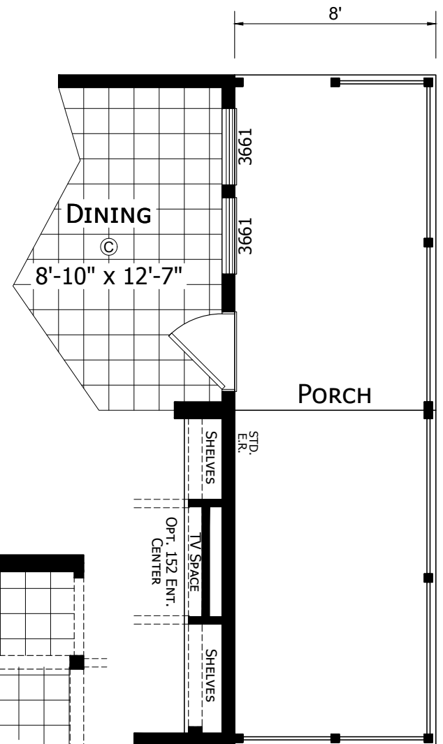
OPTIONAL PORCH
