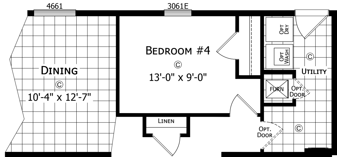
OPTIONAL BEDROOM #4
