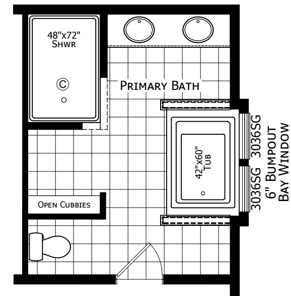
OPTIONAL SERENITY BATH
