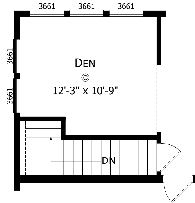
OPTIONAL STAIRWELL
