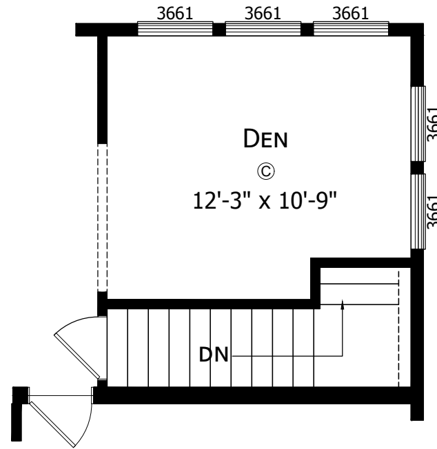
OPTIONAL STAIRWELL
