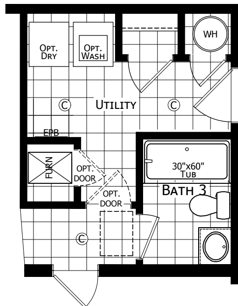
OPTIONAL BATH #3
