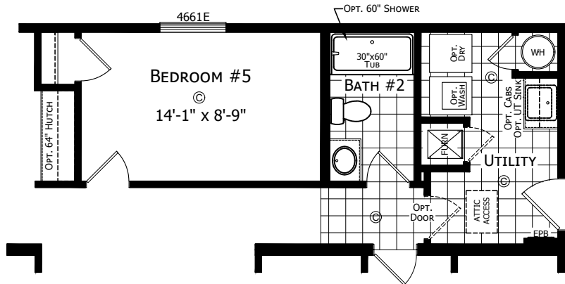
OPTIONAL BEDROOM #5
