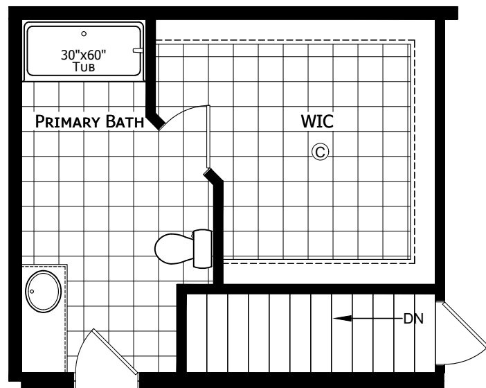
OPTIONAL STAIRWELL
