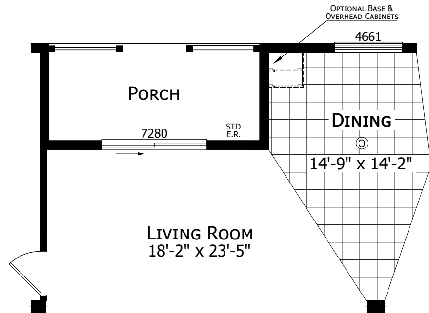
OPTIONAL PORCH
